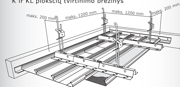
K ir KL plokščių tvirtinimo brėžinys
